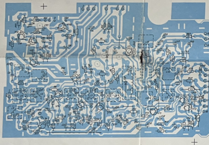
ПЛАТА ПРИЕМНОГО ТРАКТА А1
