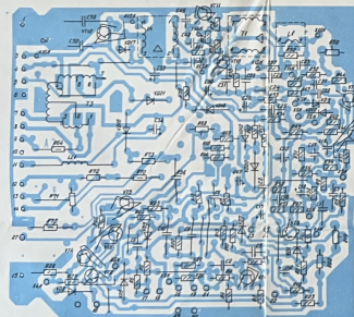
ПЛАТА РАЗВЕРТОК А2
