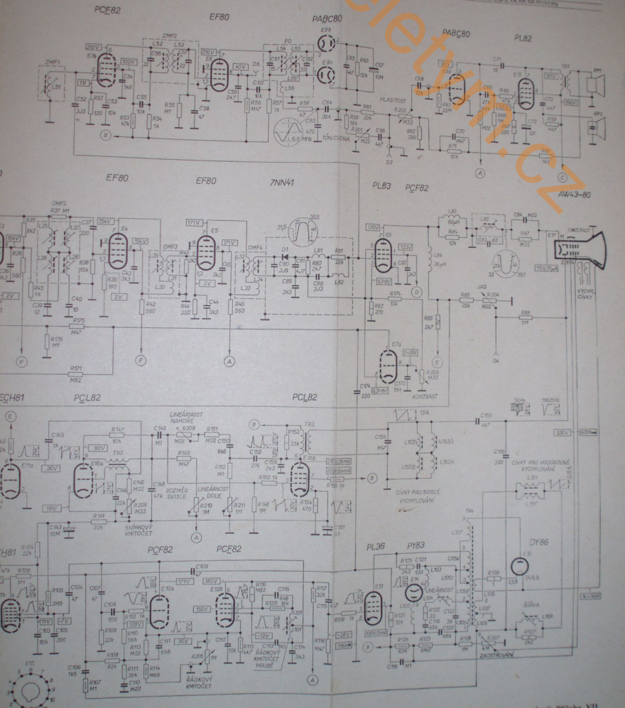
Zapojení televizního přijímače 4106U „AMETYST“ (běžné provedení) Příloha VII
