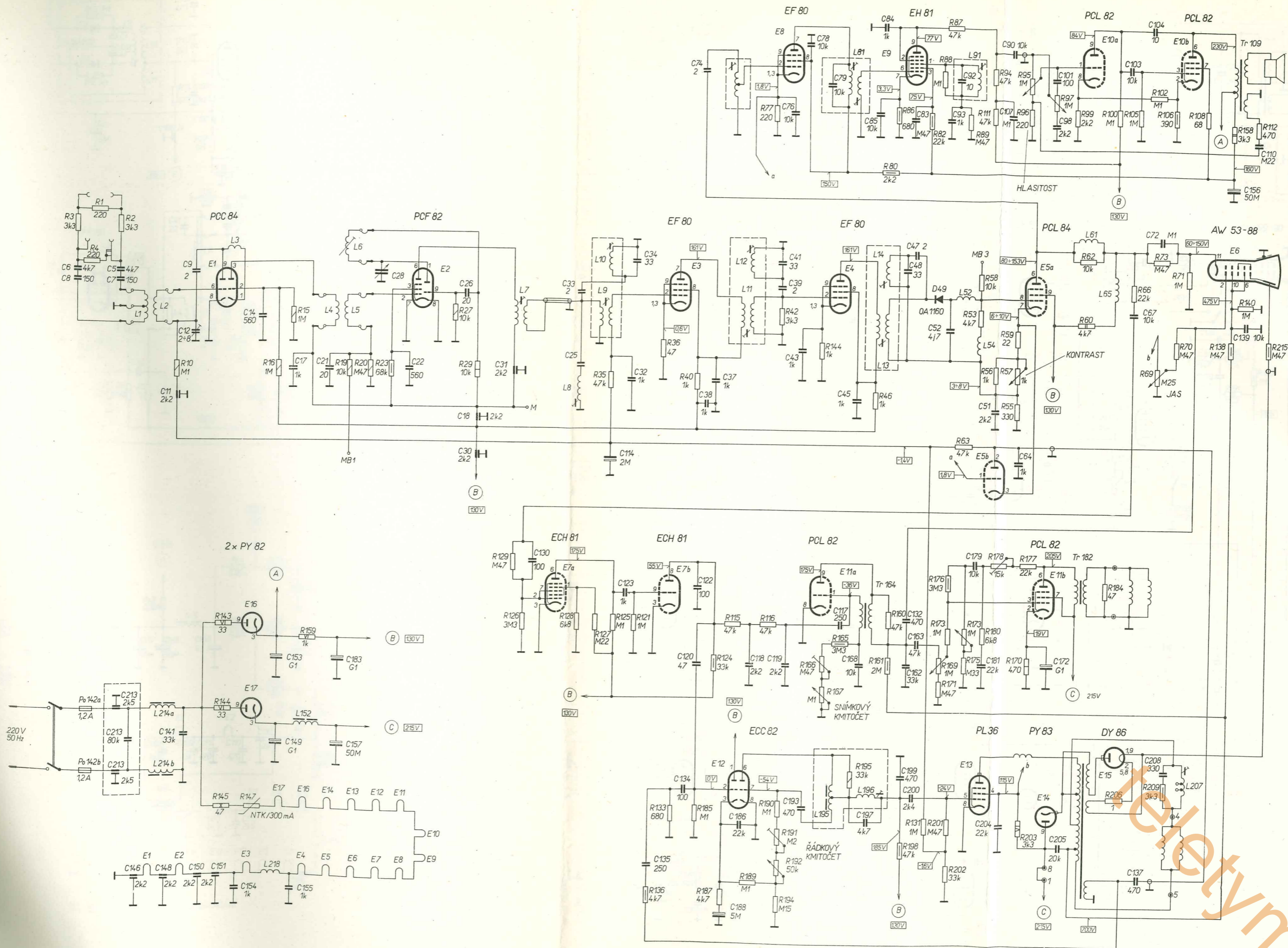
Príloha 9 — Schéma zapojení televizního přijímače ORION AT 505
