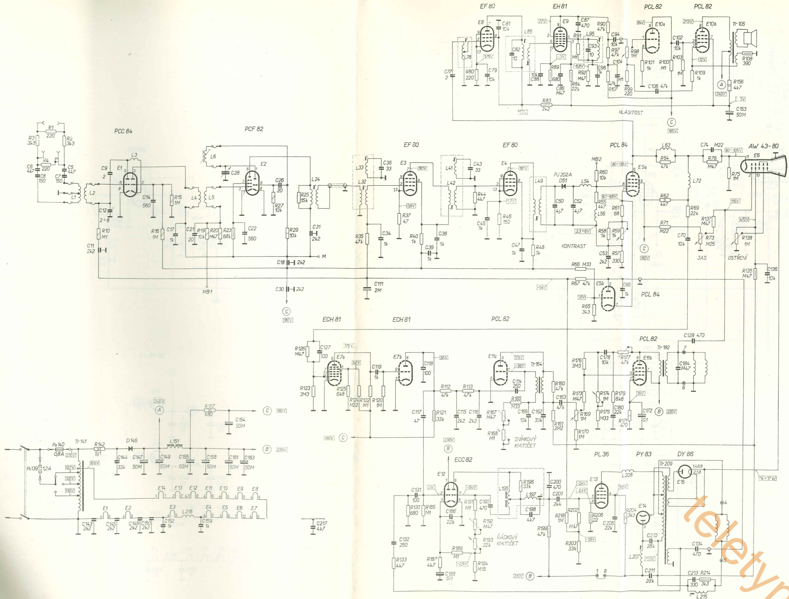
Příloha 8 — Schéma zapojení televizního přijímače ORION AT 504
