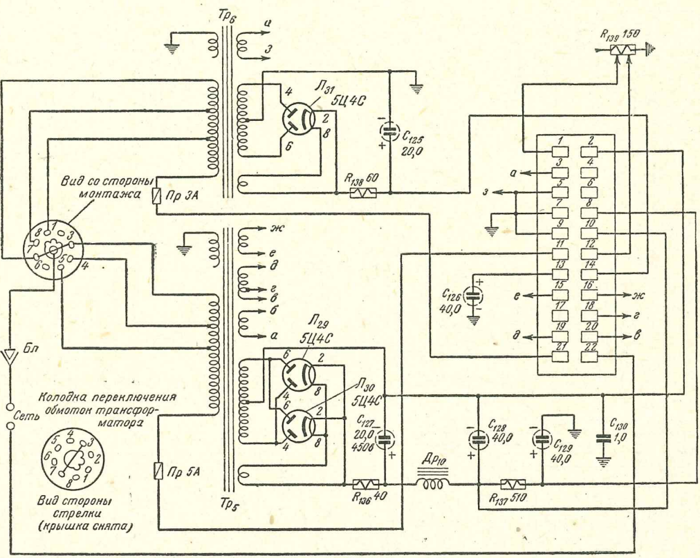
Рис. 18-11. Принципиальная схема блока низковольтных выпрямителей телевизора Т-2 «Ленинград».
