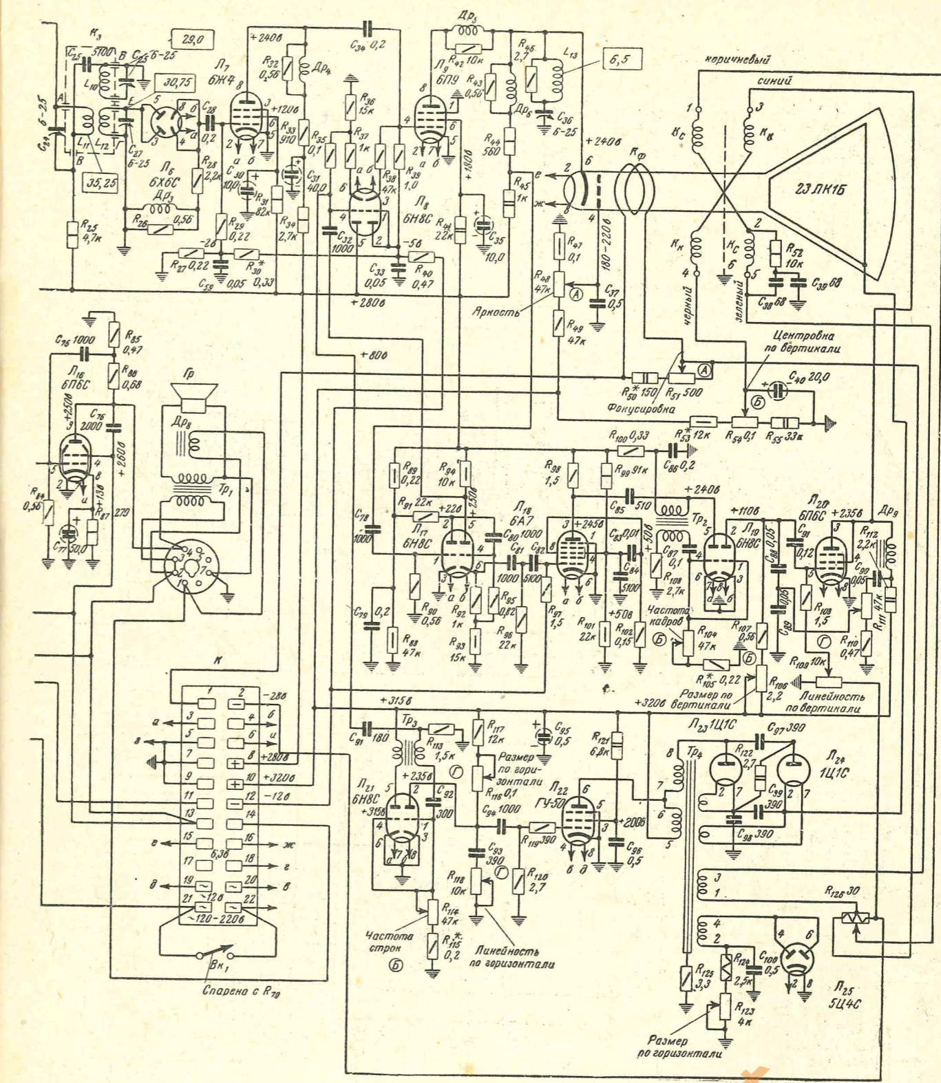
телевизора Т-2 «Ленинград». Вид на колодку К дан со стороны монтажа.
