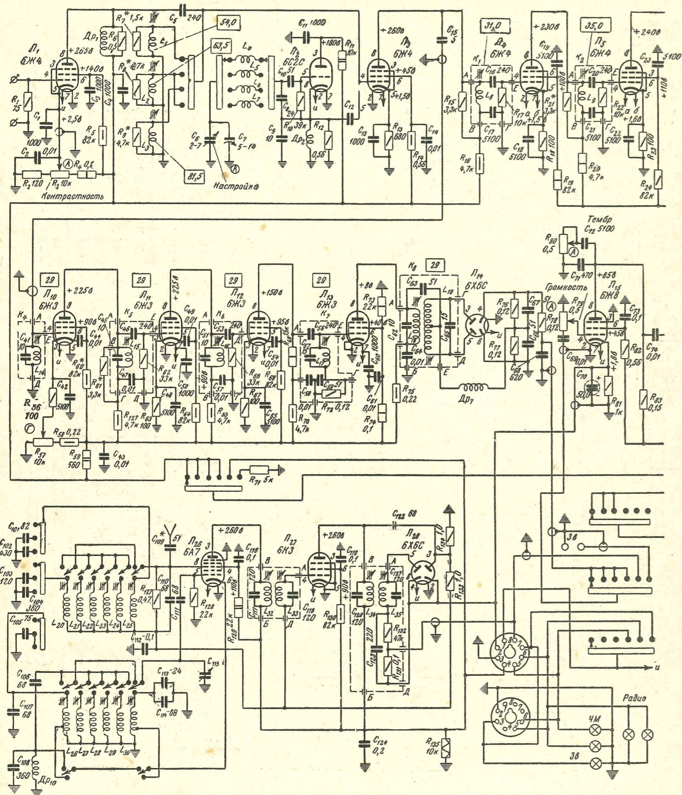
Рис. 18-4. Принципиальная схема блока приемников и блока развертки
